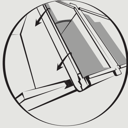
Detalhamento do encaixe do aparador
